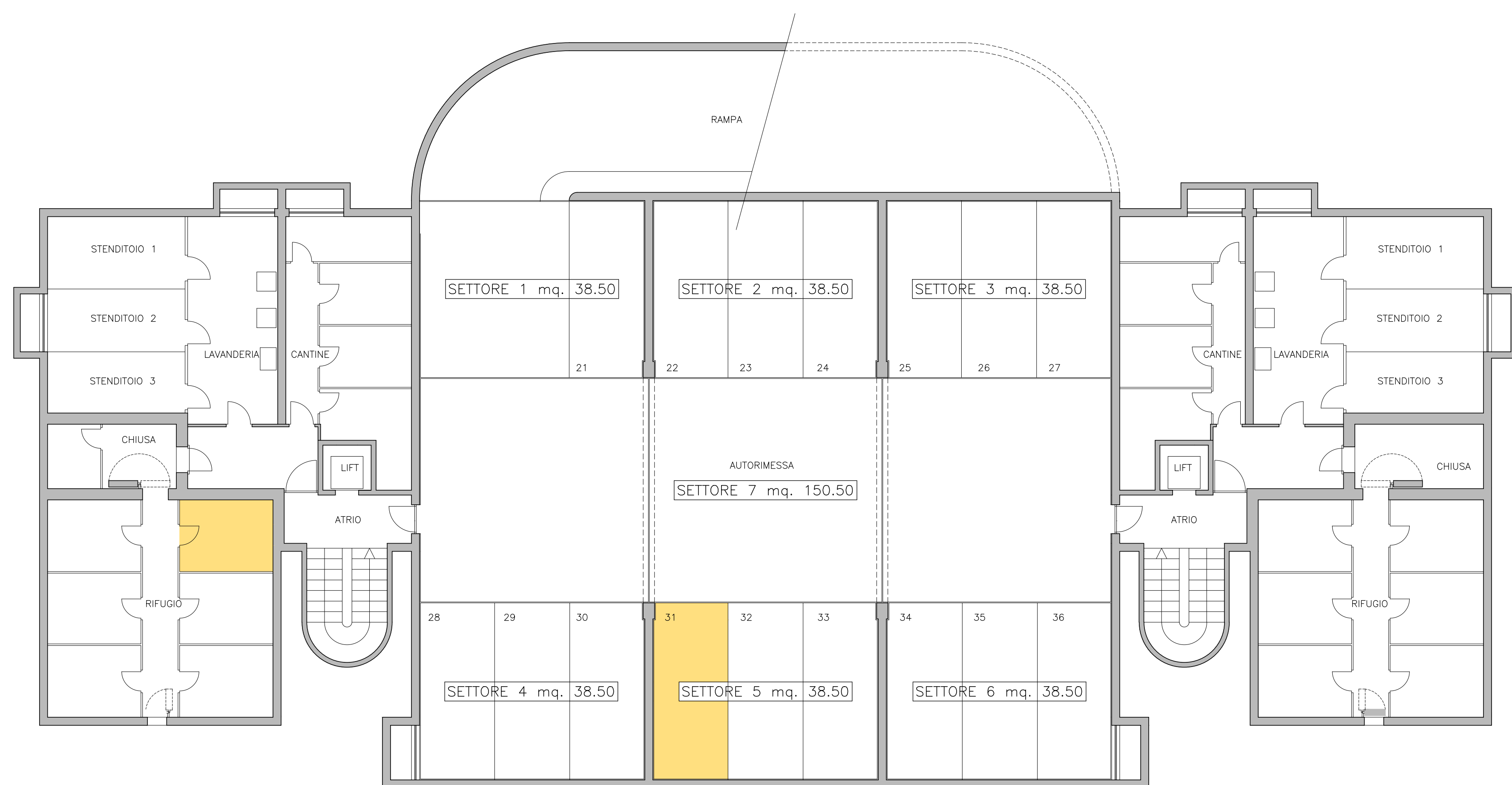
PRIMO PIANO INTERRATO
